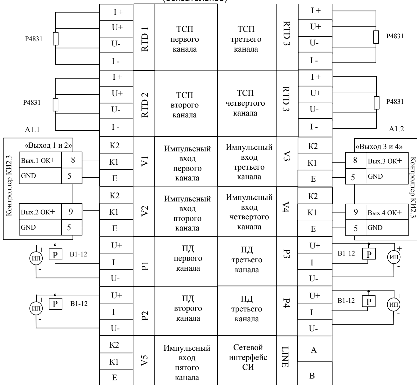
Схема подключения вычислителя ТМК-НЗ к приборам и оборудованию при его поверке (P - калибраторы тока, ТСП- термометр сопротивлений, ПД – преобразователь давления, ИП – источник питания стабилизированным напряжением U_{н}=24В I_{макс}= 50mA )
