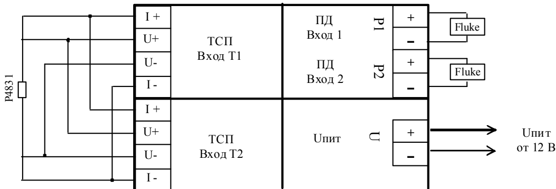
Схема подключения ТМК-Н20 к приборам и оборудованию при калибровке
