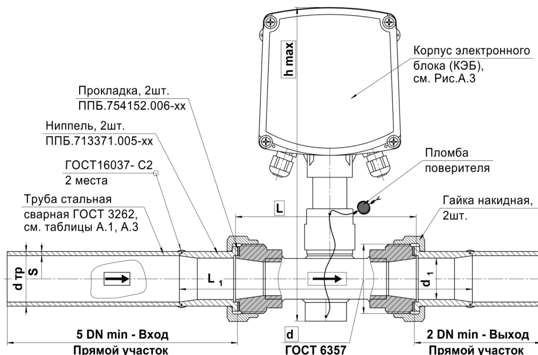
Рисунок А.1 – Габаритные и присоединительные размеры преобразователей ВПС1(2) с резьбовым присоединением DN25, 32, 40
