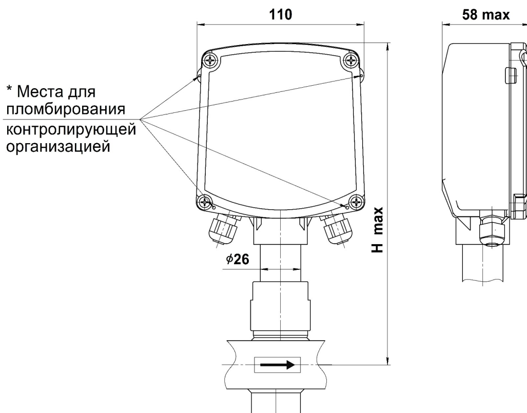
Рисунок А.3 - Габаритные размеры корпуса электронного блока для исполнений ВПС1(2) в соответствии с таблицей А.1
