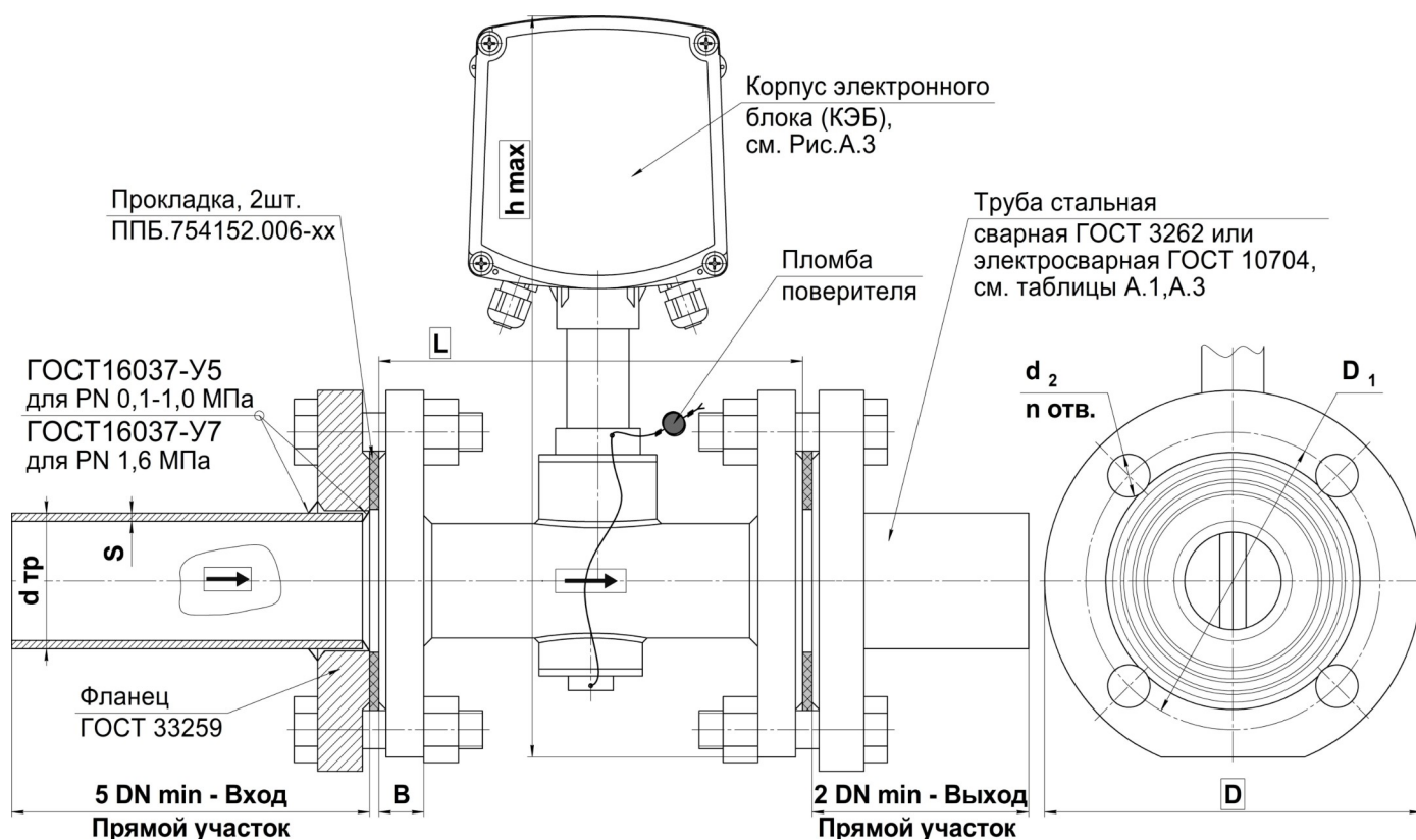
Рисунок А.2 – Габаритные и присоединительные размеры преобразователей ВПС1(2) с фланцевым присоединением DN50, 65, 80, 100, 150
