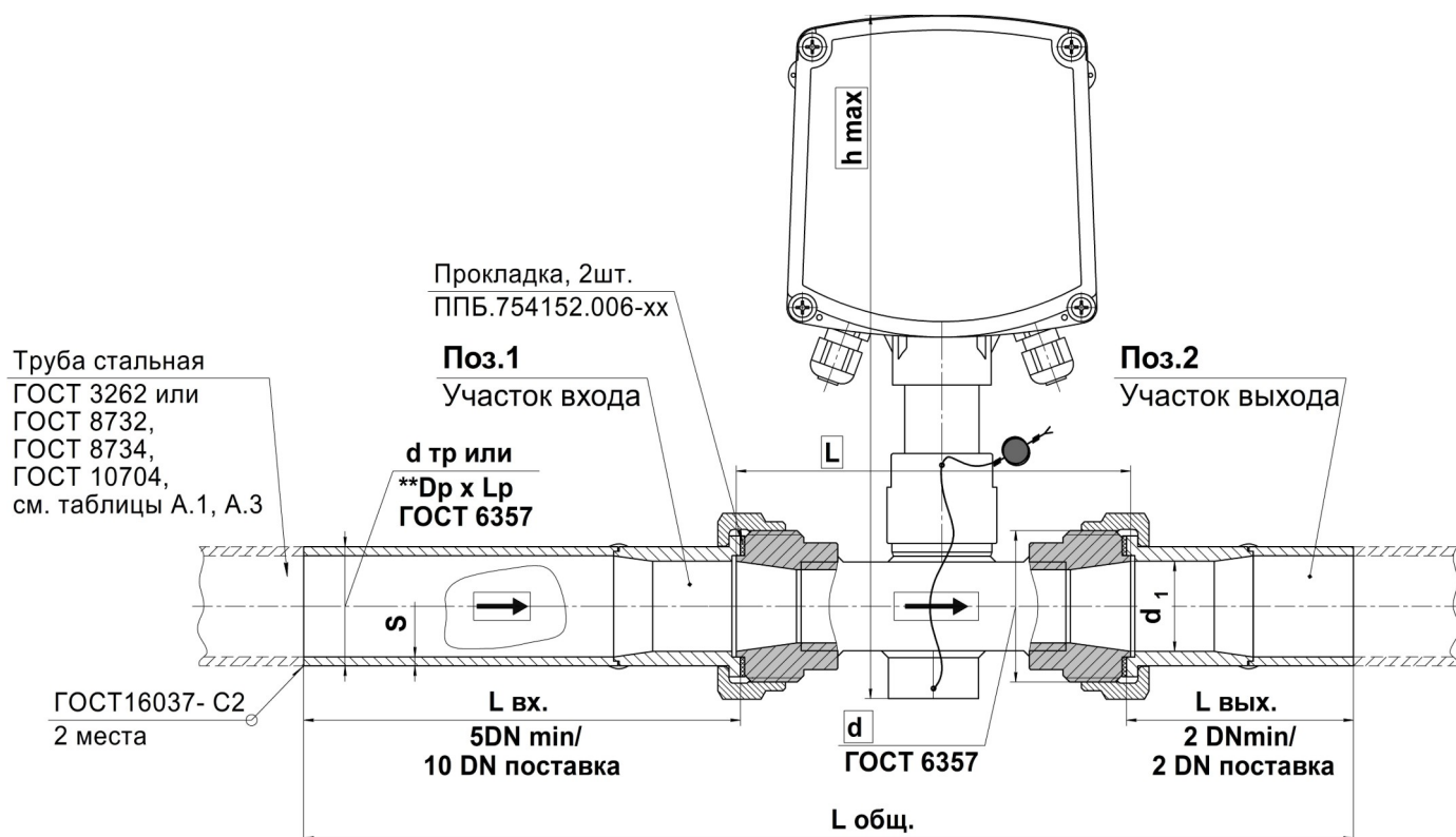
Рисунок А.4 – Поставка преобразователей с комплектом монтажных частей КМЧ ВПС №2 (в соответствии с таблицей А.2)
