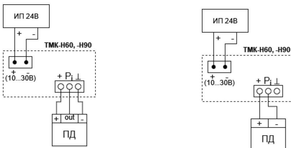
Трехпроводная схема с внутренним питанием ПД
