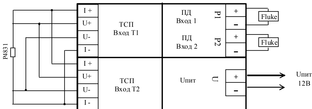
Схема подключения ТМК-Н120 к приборам и оборудованию при калибровке
