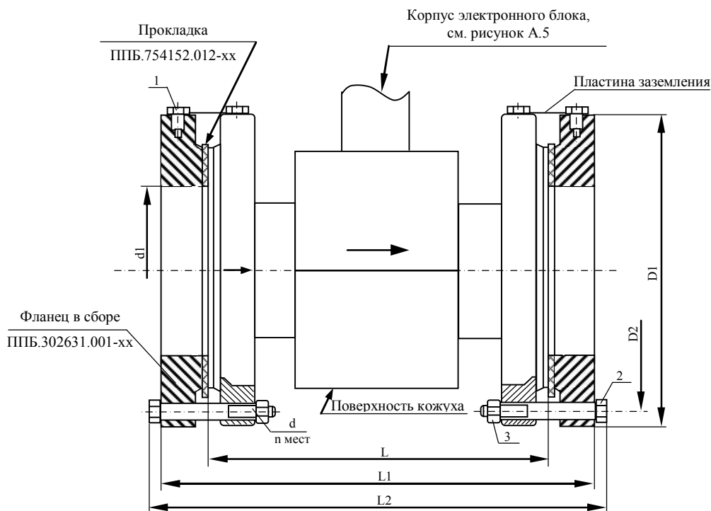
Рисунок А.1а – Доставка фланцевых ПР исп.МФ-5.2.1 с комплектом монтажных частей КМЧ МФ №3
