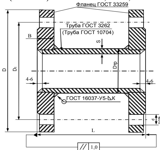
Рисунок А.10 – Макет 1 – фланцевый, ПР МФ-2, МФ-5
