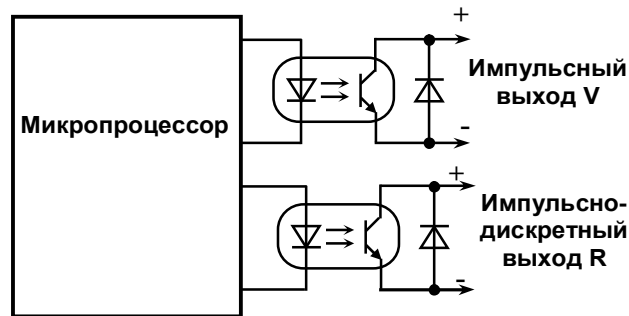
Рисунок 3.3 - Организация выходов исп. ИС.МФ-Ч (плата ПР)
