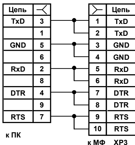
Розетка DB-9F
