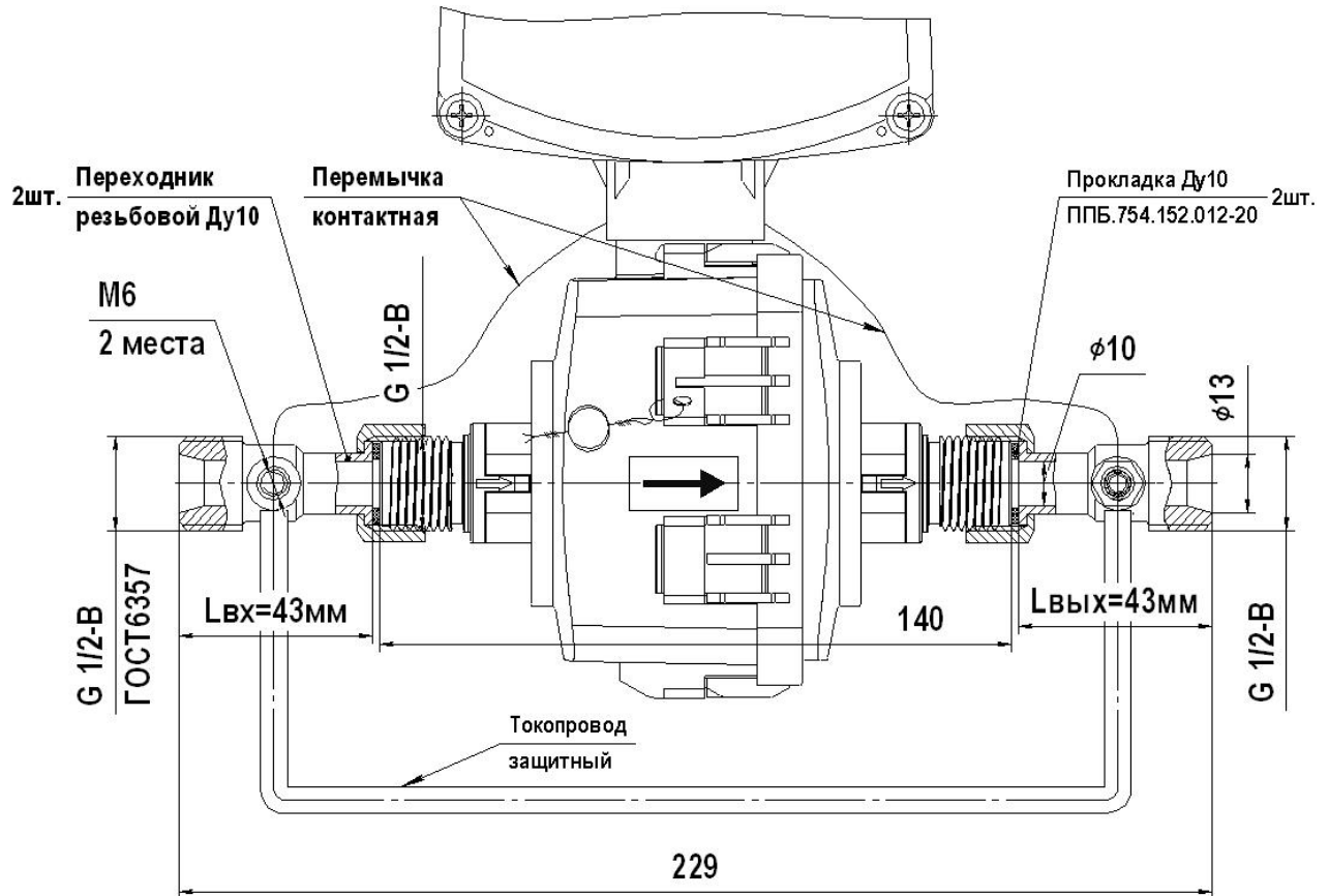
Рисунок А.8б – Габаритные размеры ПР МФ исп. ИС.МФ-10.2.1 DN10 с комплектом монтажных частей: КМЧ МФ №10 (резьбовой, с гайкой накладной)
