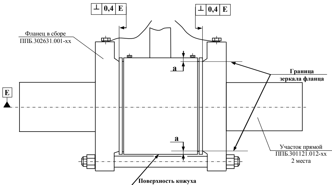
Рисунок А.13 – Требования к точности установки фланцев прямых участков
