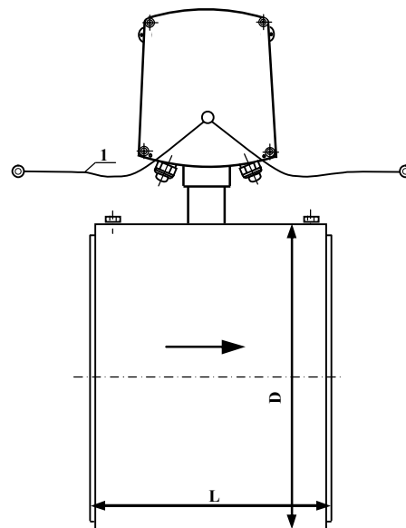
Рисунок А.4 – Поставка бесфланцевых ПР МФ-2.2.х без КМЧ
