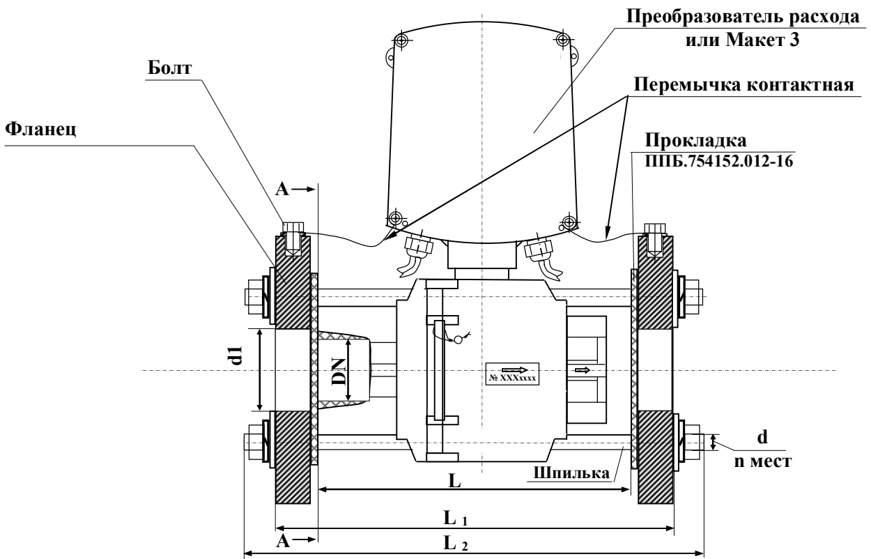
Габаритные и присоединительные размеры в соответствии с таблицей А.9.
