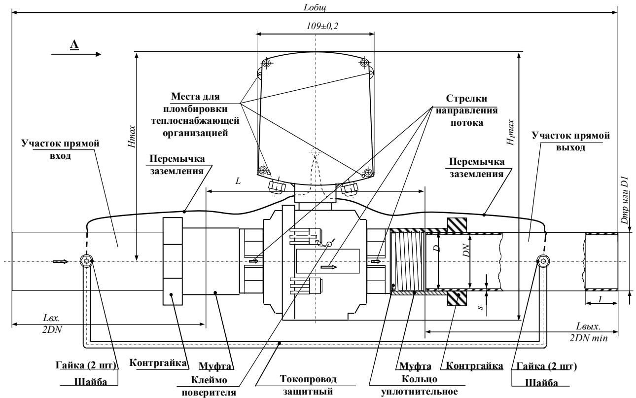
Рисунок А.8а– Габаритные размеры ПР исп. МФ-10.2.1 DN10, DN20, DN32 с комплектом монтажных частей : КМЧ МФ №6 (приварной) или КМЧ МФ №7 (резьбовой)
