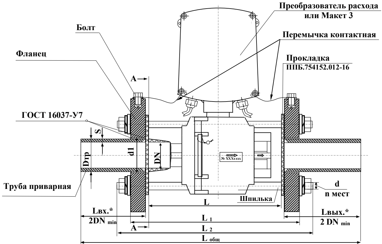
Рисунок А.96 – Габаритные размеры бесфланцевых ПР МФ-10.2.1- 50 с комплектом монтажных частей КМЧ МФ № 9 (фланцы с приваренной трубой)
