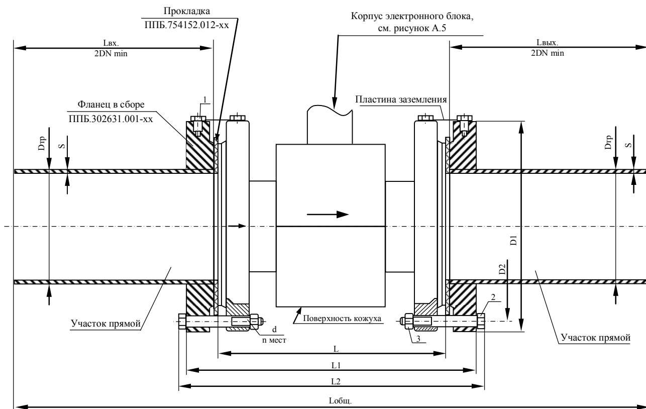
Рисунок А.16 – Поставка фланцевых ПР исп. МФ-5.2.1 с комплектом монтажных частей КМЧ МФ №4 с прямыми участками трубопроводов
