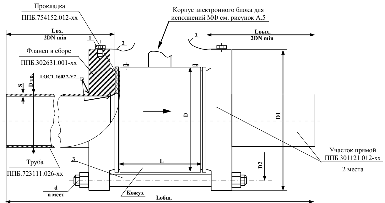
Рисунок А.2 – Поставка бесфланцевых ПР исп. МФ-2.2.1 с комплектом монтажных частей КМЧ МФ №2 с прямыми участками трубопровода
