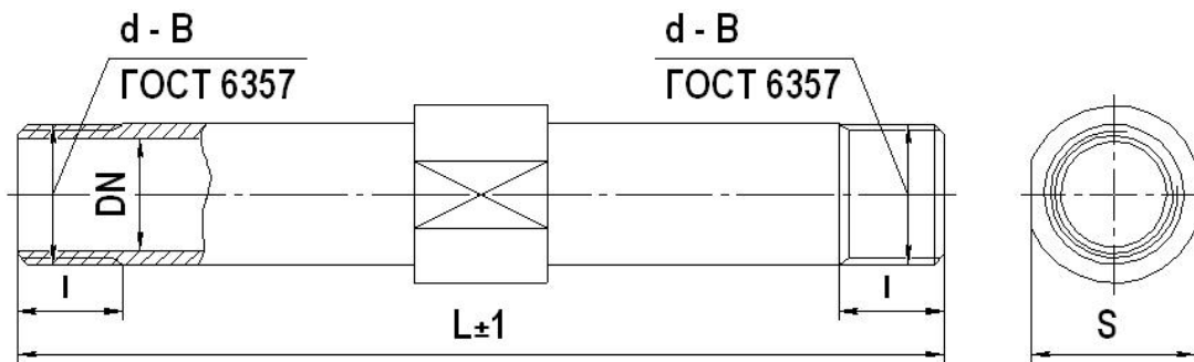
Рисунок А.11 – Макет 2 – резьбовой пластиковый ПР исп. МФ-10.2.1 DN10, DN20, DN32
