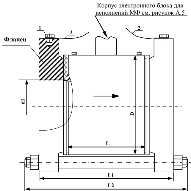
Рисунок А.3 – Поставка бесфланцевых ПР МФ-2.2.х с фланцами, КМЧ МФ №1
